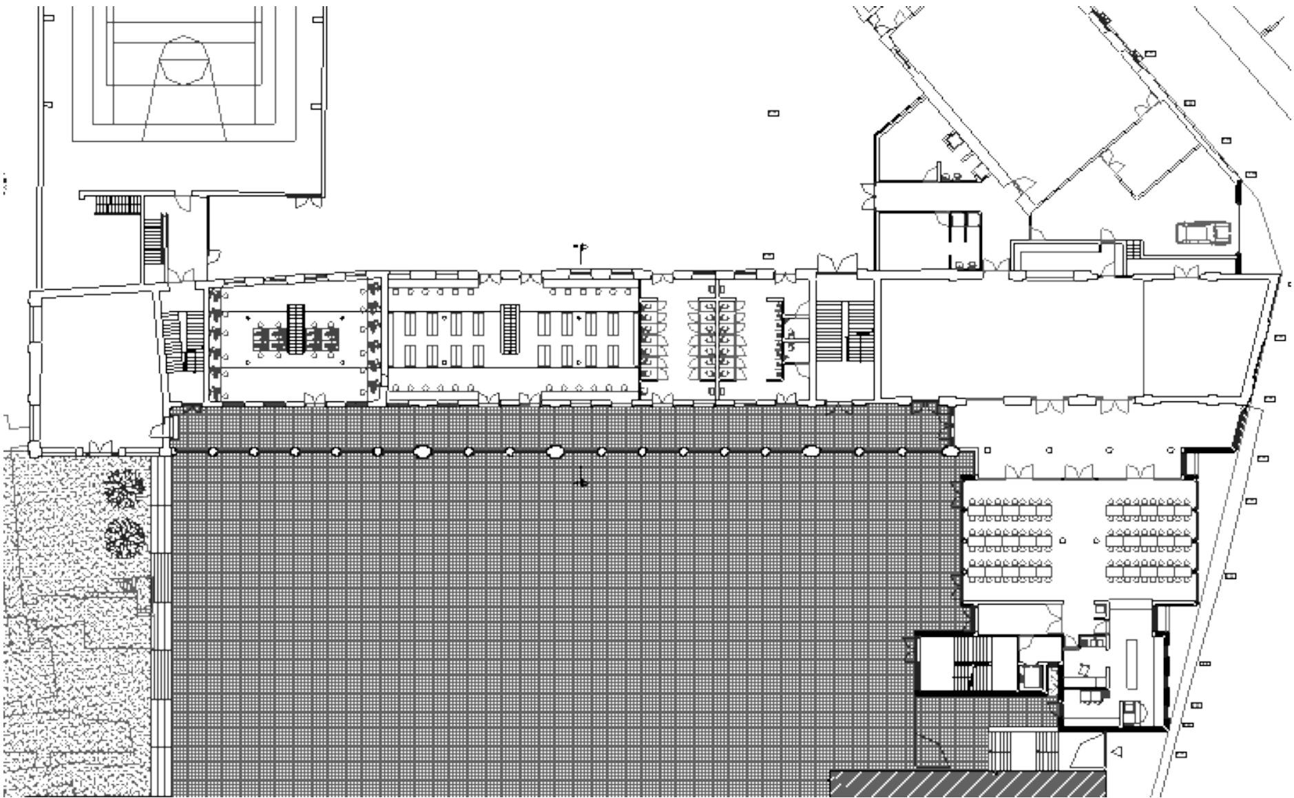
Vue en plan du rez-de-chaussée
