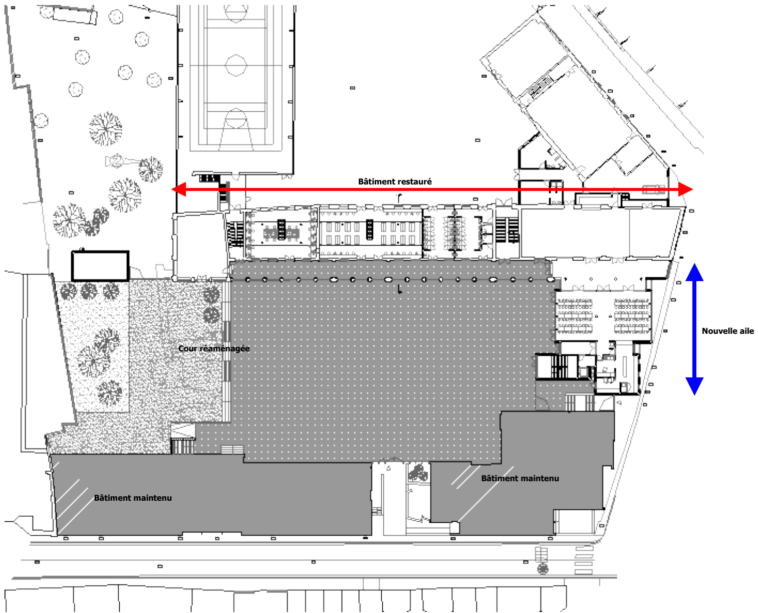
Implantation projetée – vue en plan du rez-de-chaussée
